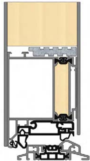
W82 RQS Flügelüberdeckung beidseitig Blendrahmen abgerundet
