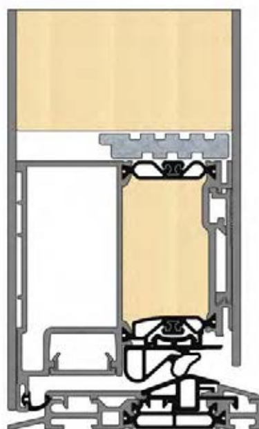
W92 QS Flügelüberdeckung beidseitig
