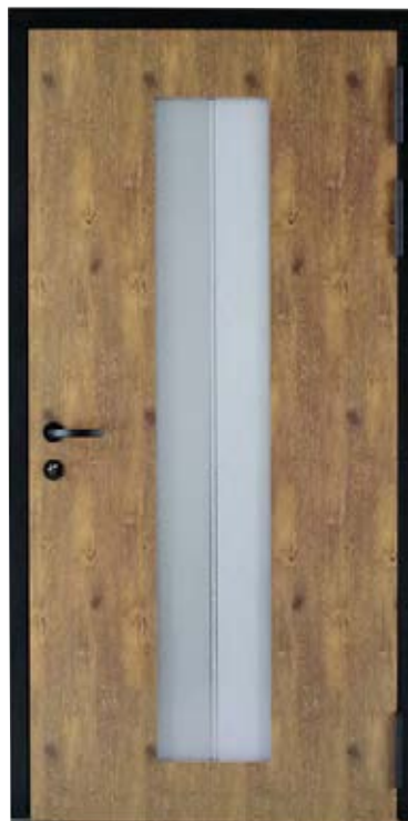
LAN 333 Farbe: Türrahmen ST 9005 schwarz, Türfüllung Holzoptik Eiche Brettholz senkrecht D 131 mit Nutenfräsung außen Applikation oben/unten Struktur waagrecht Glastyp: 333.8014 Klarglas halbseitig mattiert mit Dekorkante 3-D-Effekt (Dreifachverglasung erforderlich) Griff: HE 116 schwarz (600 mm) halbrund mögliche Innenansicht mit Flügelüberdeckung, Profil ohne Aufschlagdichtung, Rollentürbänder schwarz Innengriff: S 5405 schwarz Feinstruktur
